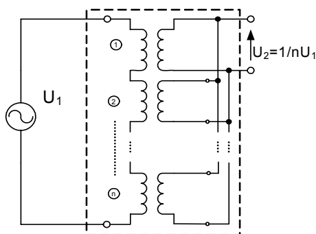
Fig. 16. n-module
